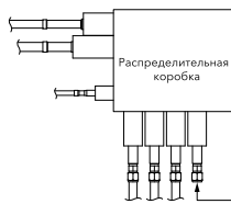
Используйте три соединительных порта. Пример. Если одно соединение трубопроводов не используется, убедитесь в том, что установленная изготовителем глухая конусная гайка затянута (на стороне газа и жидкости).
