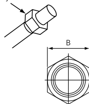
Размер конусной гайки В (мм)
